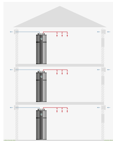
Wohnungslüftung mit Brauchwarmwasserbereitung im Mehrfamilienhaus
