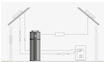
Kombi-Brauchwarmwasser-Wärmepumpe
