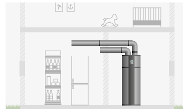
Brauchwarmwasserbereitung, Abwärmeebenutzung im Umluftbetrieb
